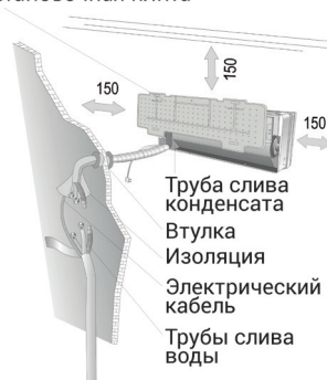
Установочная плита
