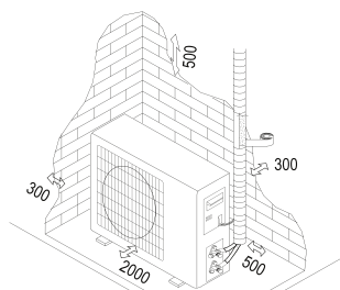
Минимальное пространство (мм) для монтажа внешнего блока
